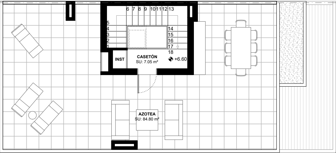
PLANTA CAJETÓN
