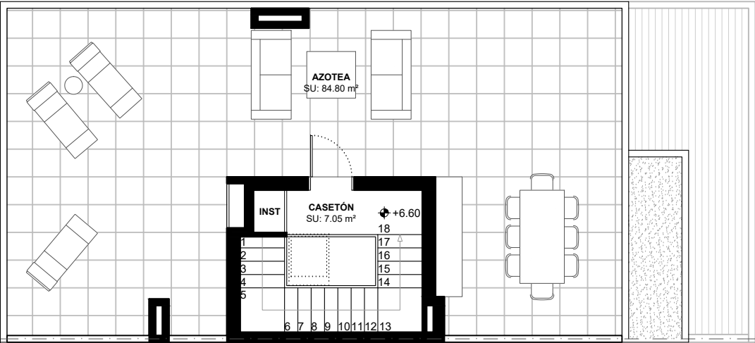
PLANTA CASETÓN
