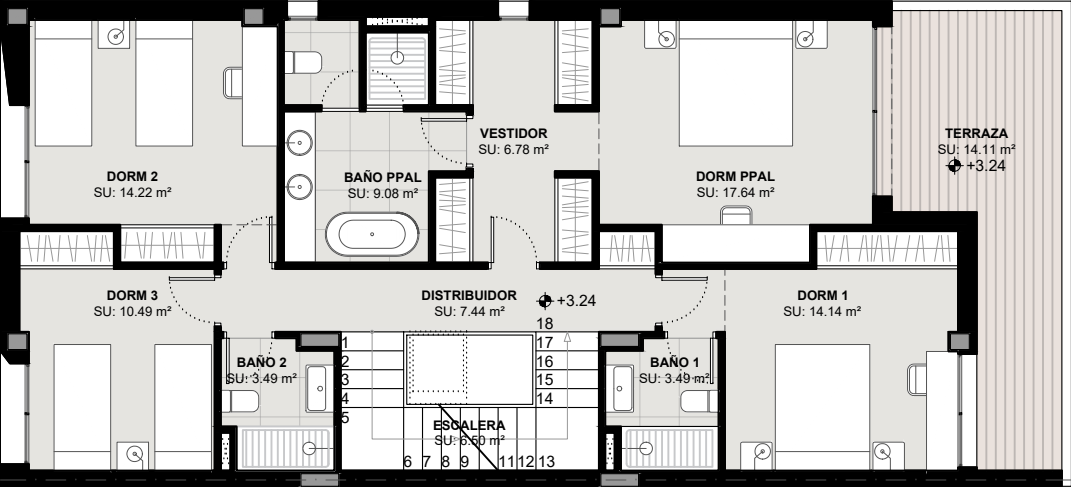
PLANTA ALTA
