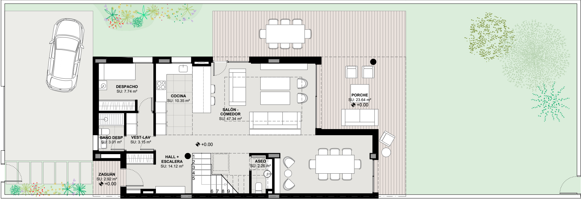
PLANTA BAJA
